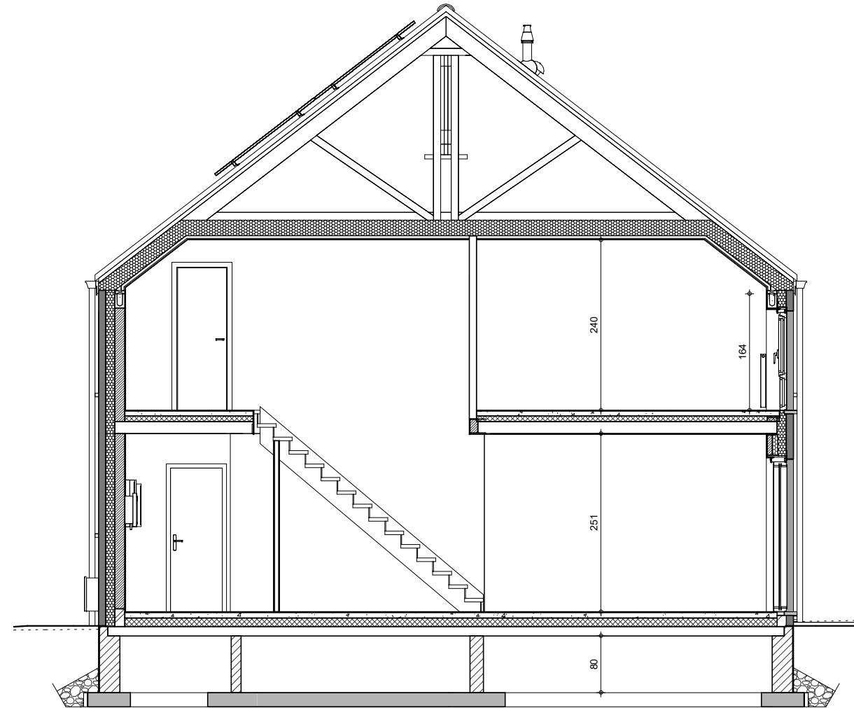
COUPE A-A LOT 61
