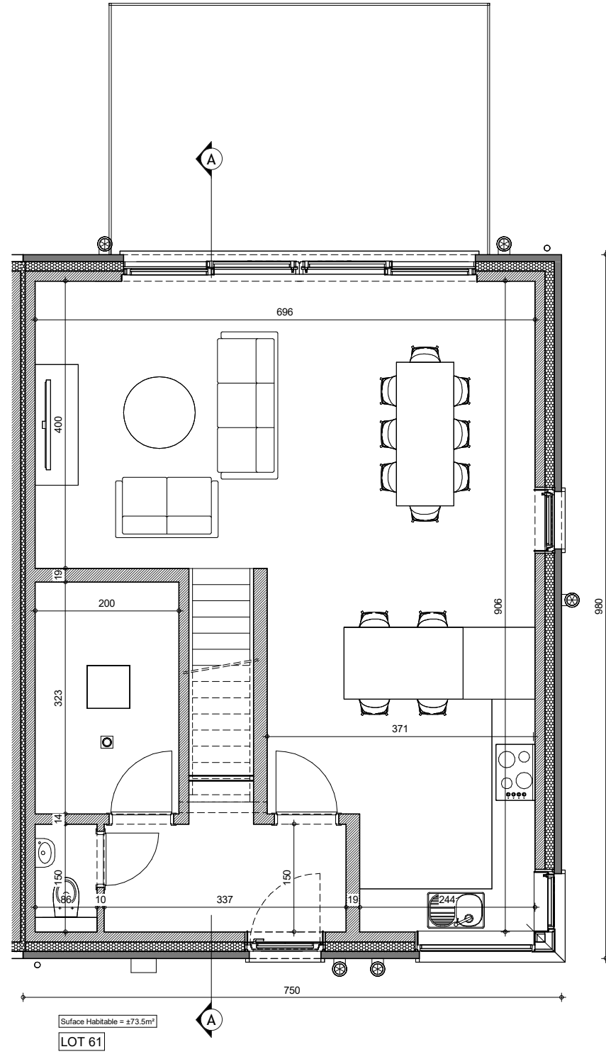
REZ-DE-CHAUSSEE
