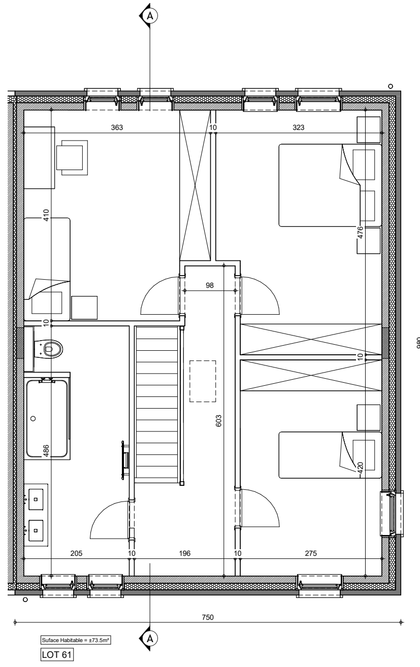
ETAGE
