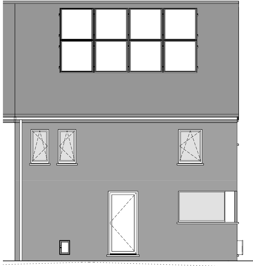
FACADE AVANT
